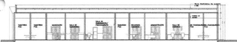
4 CORTE 04 SECC 4-5
