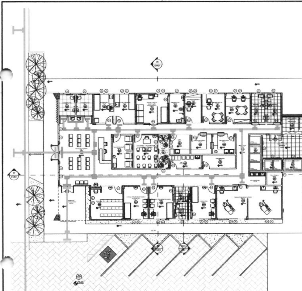
● PLANTA BAIXA ESC. 1/100
