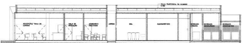
2 CORTE 02 SECC 2-3
