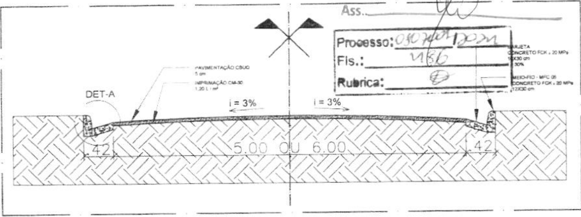
01 PERIL TRANSVERSAL ESQUEMÁTICO 01 ESCALA 1:50
