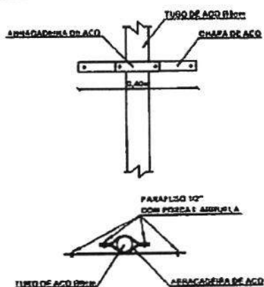
DETALHE DE FIXAÇÃO DO TUBO NA PLACA
