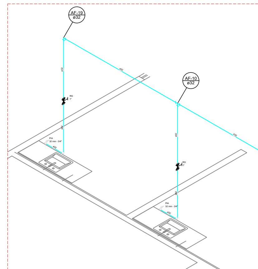
ISOMÉTRICO – H8 ESC. S/ESC
