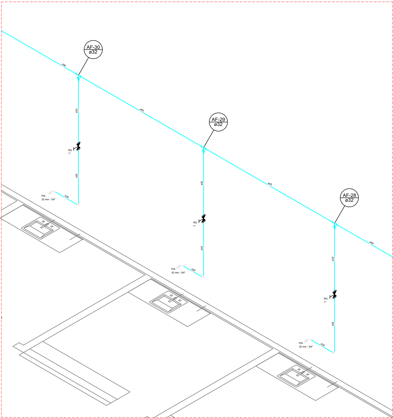
ISOMÉTRICO — H15 ESC. S/ESC
