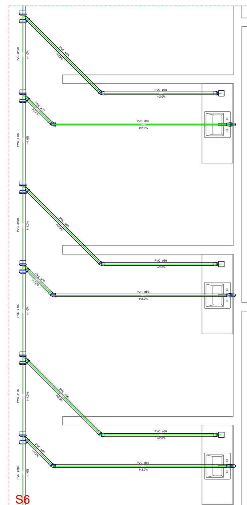
DETALHE S6
