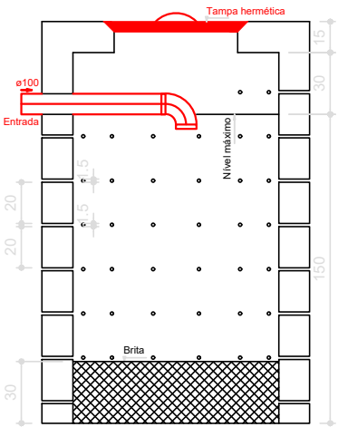
SUMIDOURO CORTE - ESC. 1:25
