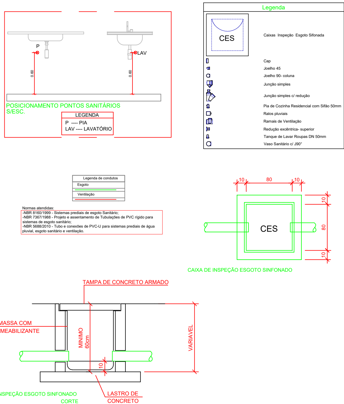
DETALHE S1
