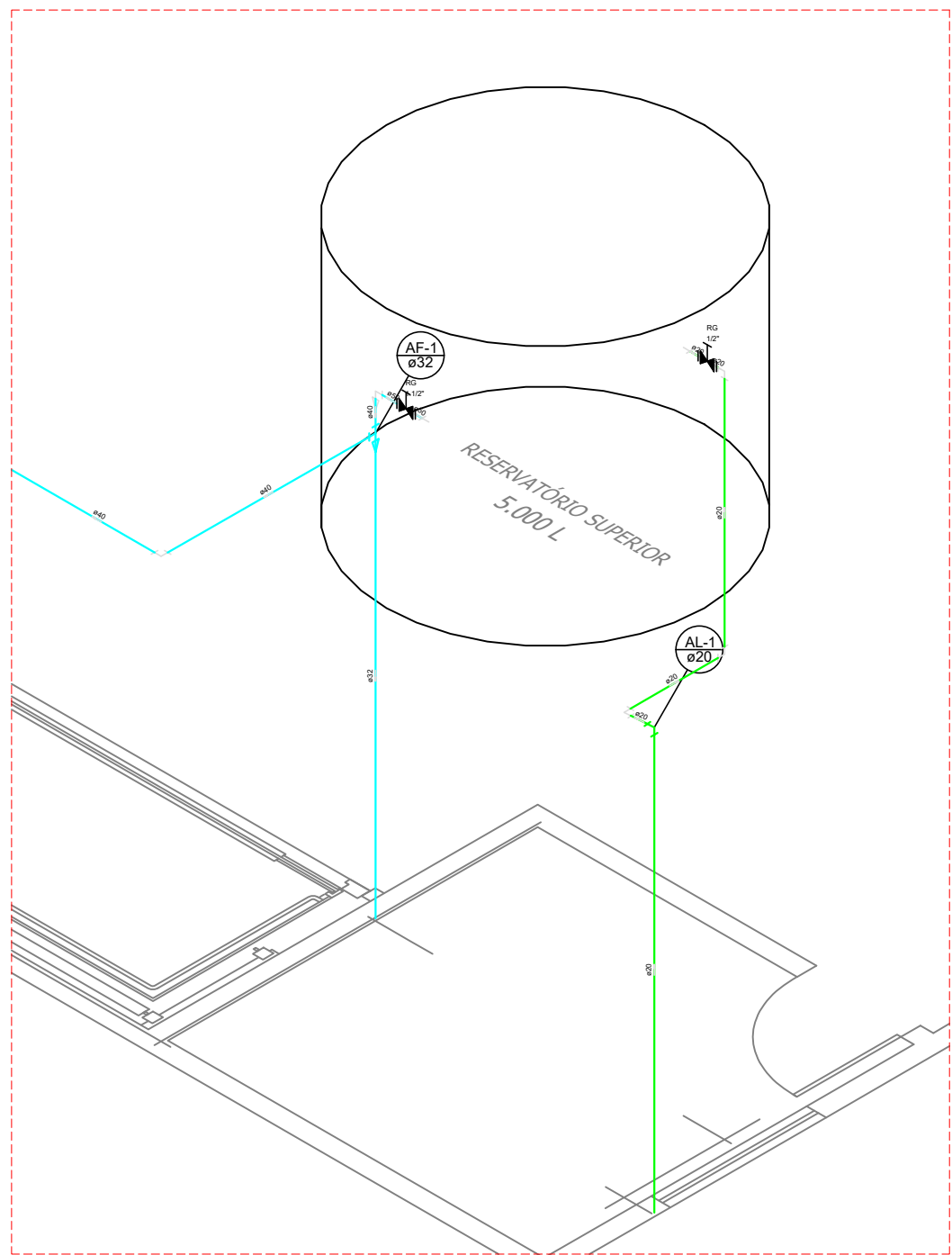
ISOMÉTRICO — H10 ESC. S/ESC
