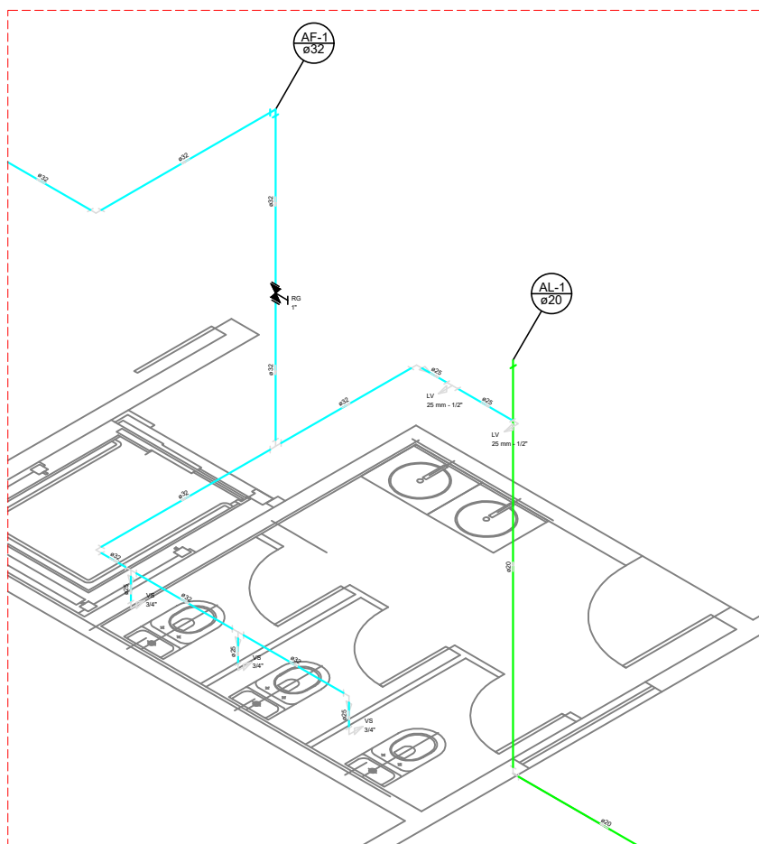
ISOMÉTRICO – H2 ESC. S/ESC
