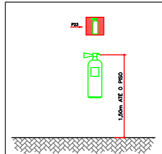
DET-3 EXTINTOR 1/100
