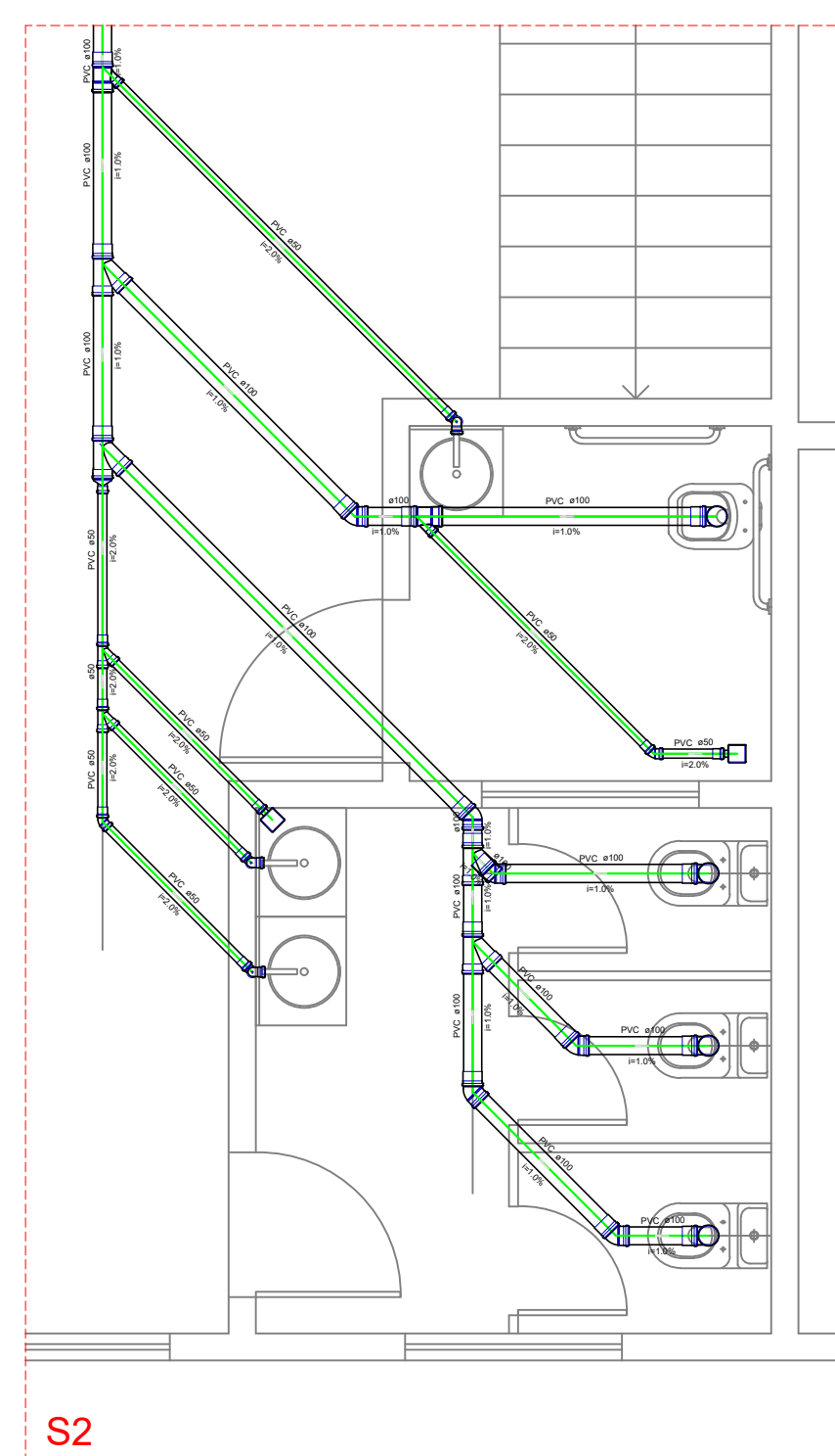
DETALHE S2
