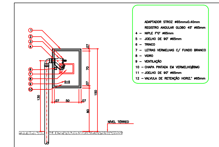
1/ESQ. CAIXA DE INCENDIO
