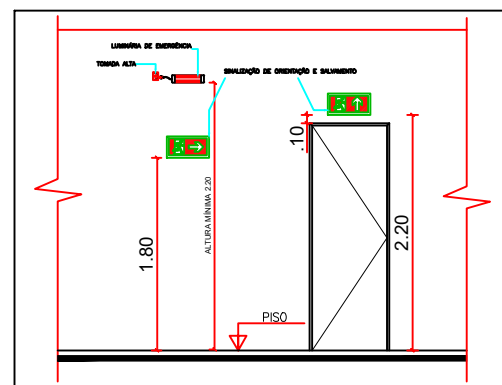
DET-2 SINALIZAÇÃO 1/100
