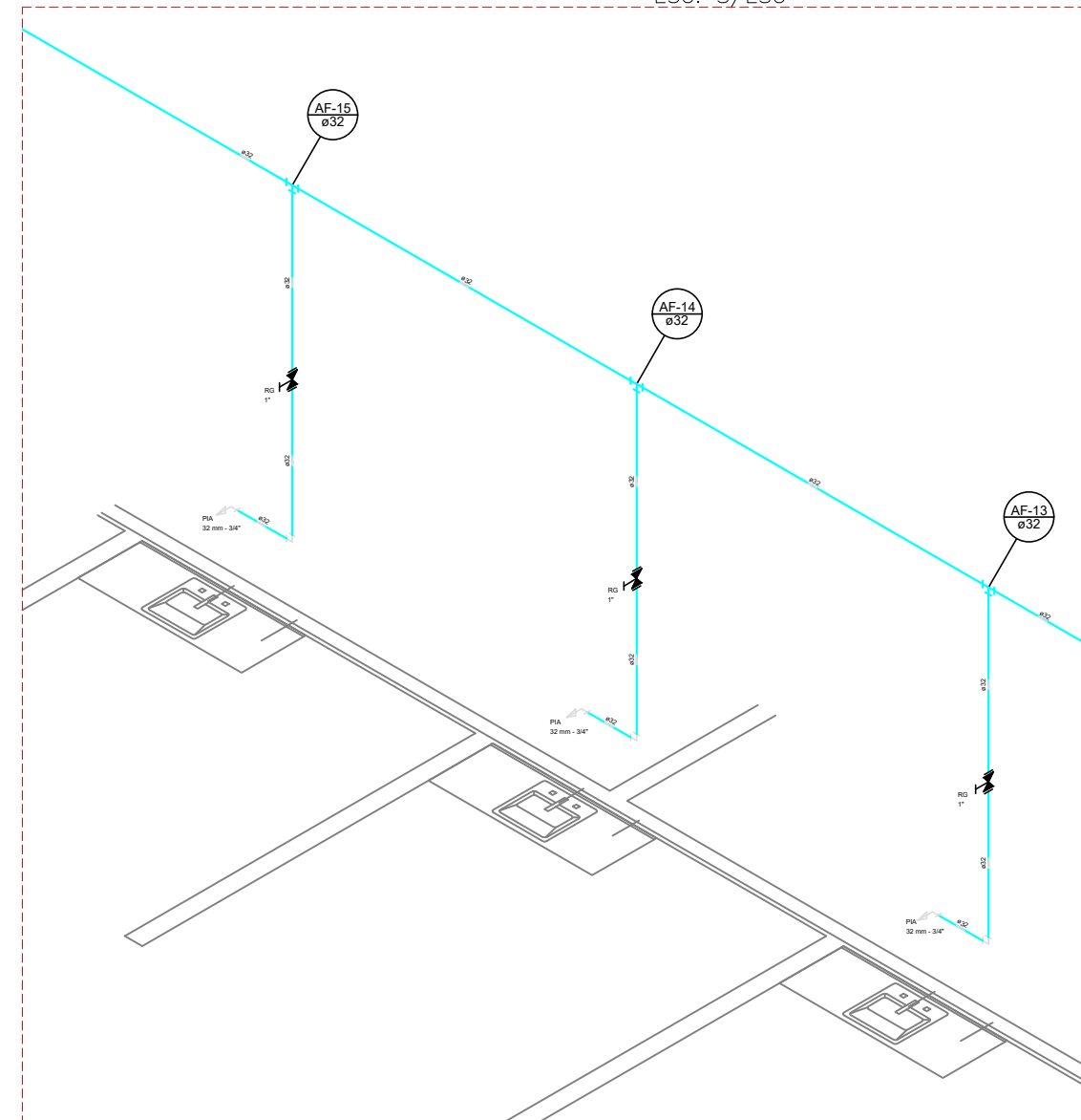
ISOMÉTRICO – H7 ESC. S/ESC
