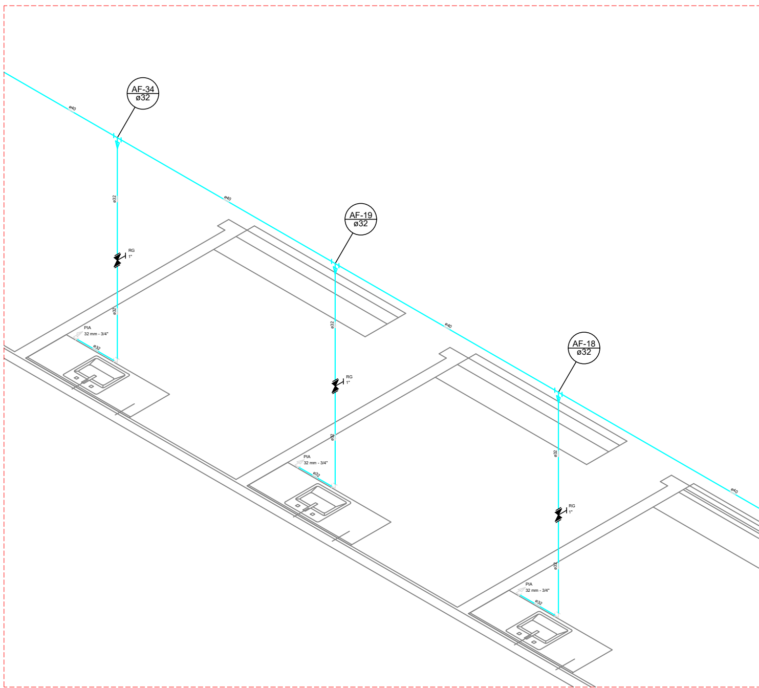
ISOMÉTRICO — H12 ESC. S/ESC
