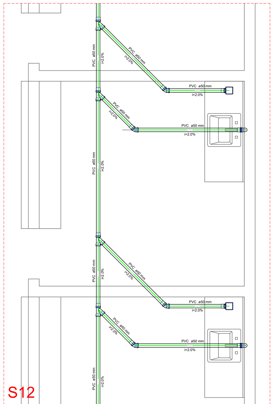
DETALHE S1
