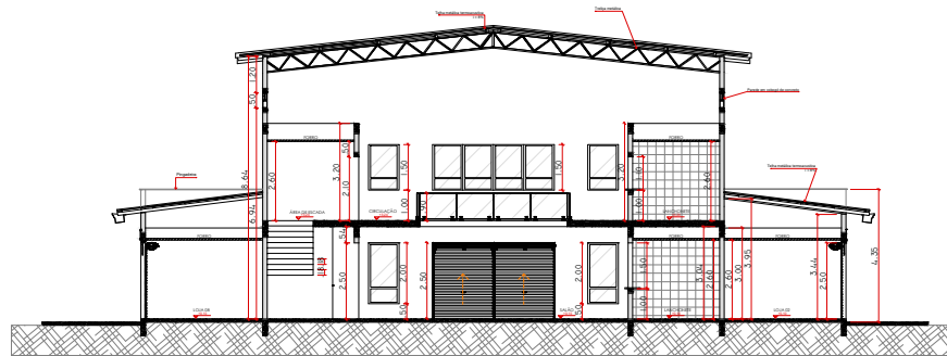
17 CORTE TRANSVERSAL AA 1:100
