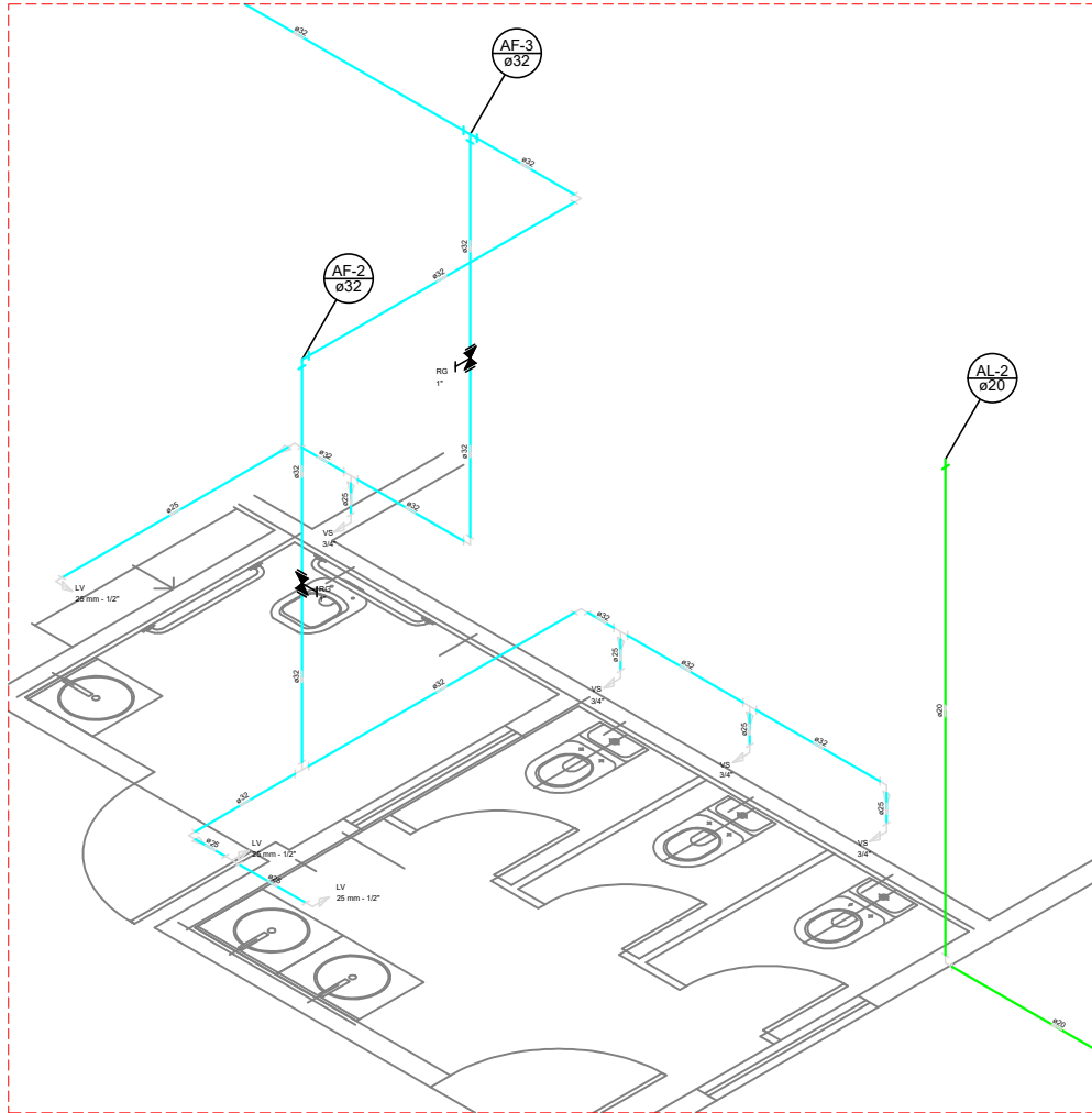
ISOMÉTRICO – H3 ESC. S/ESC
