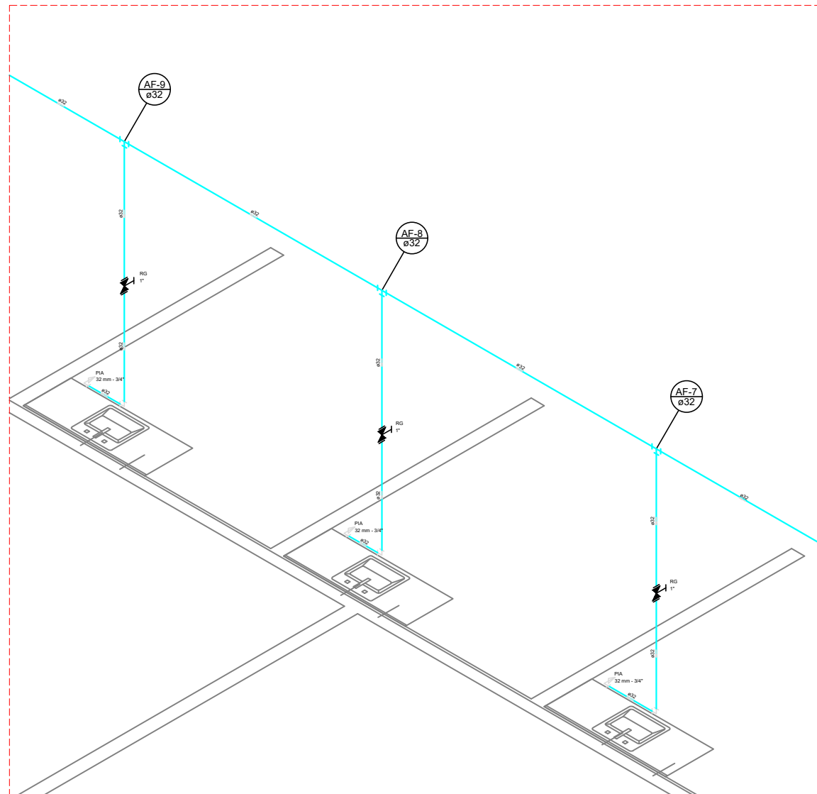
ISOMÉTRICO – H6 ESC. S/ESC
