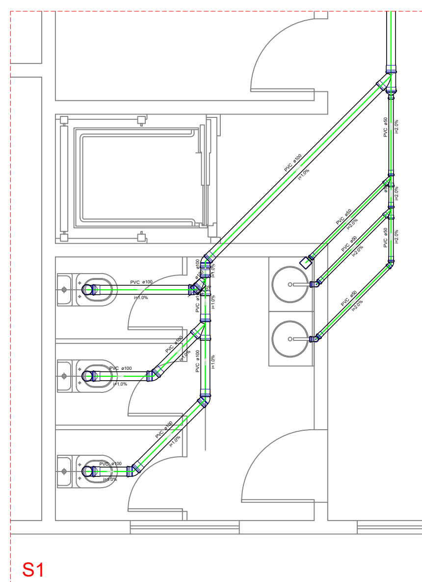
DETALHE S1
