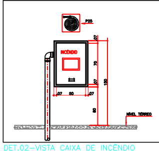
DET-4 CAIXA DE INCÊNDIO 1/100
