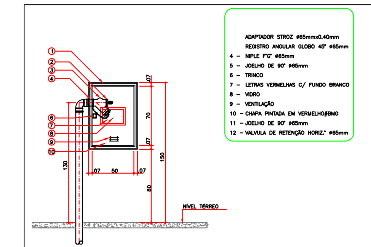
DET-1 CAIXA DE INCÊNDIO 1/100
