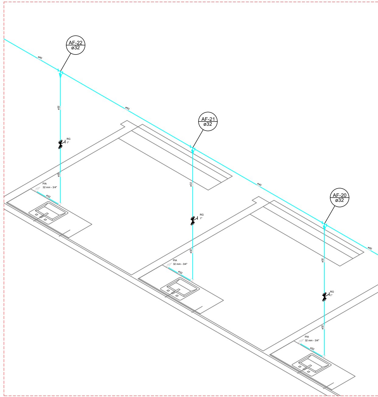
ISOMÉTRICO — H14 ESC. S/ESC
