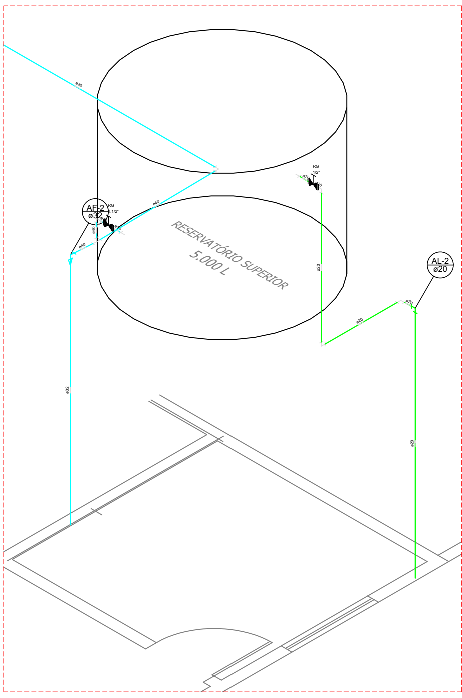
ISOMÉTRICO — H11 ESC. S/ESC
