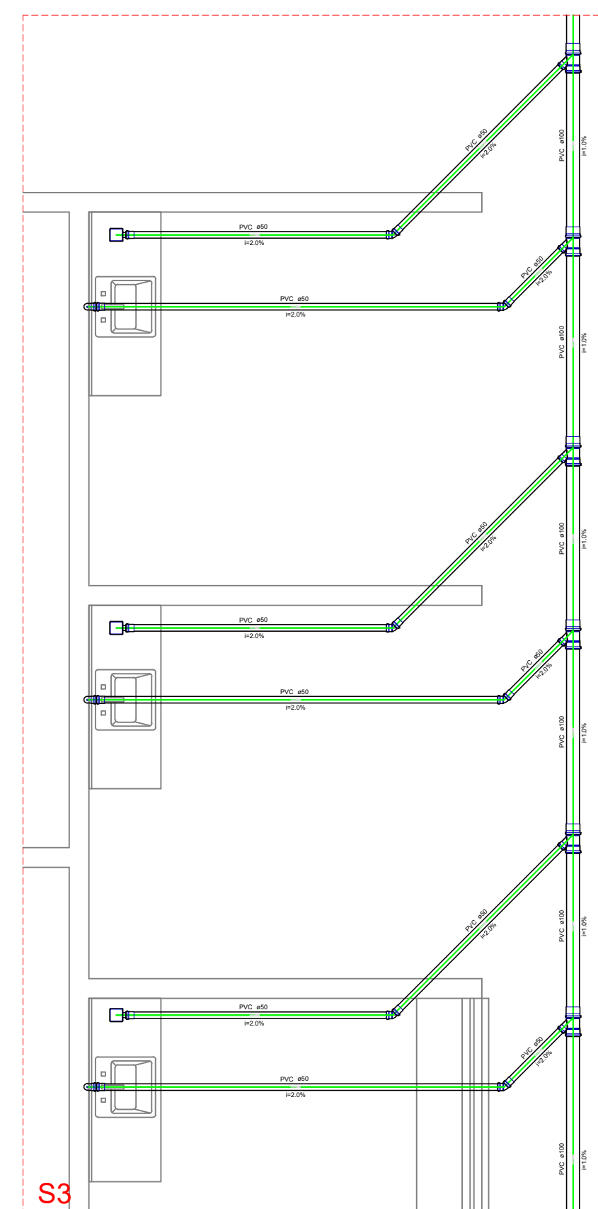
DETALHE S3
