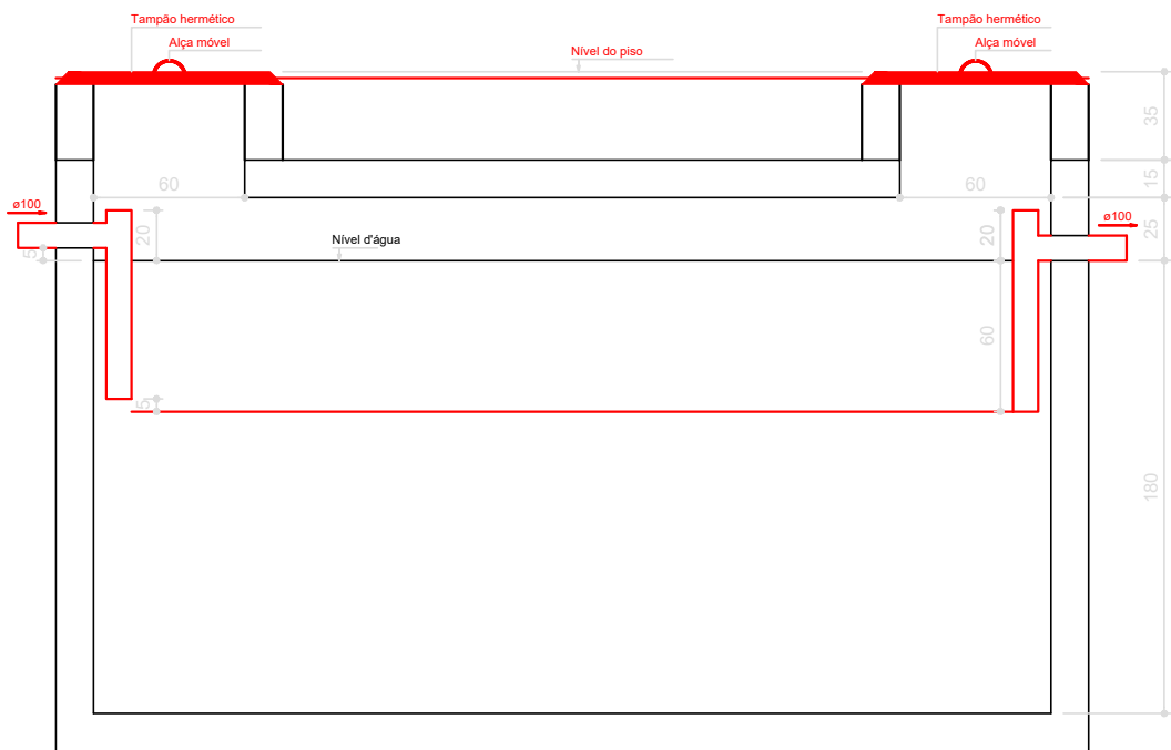
TANQUE SÉPTICO CORTE - ESC. 1:25
