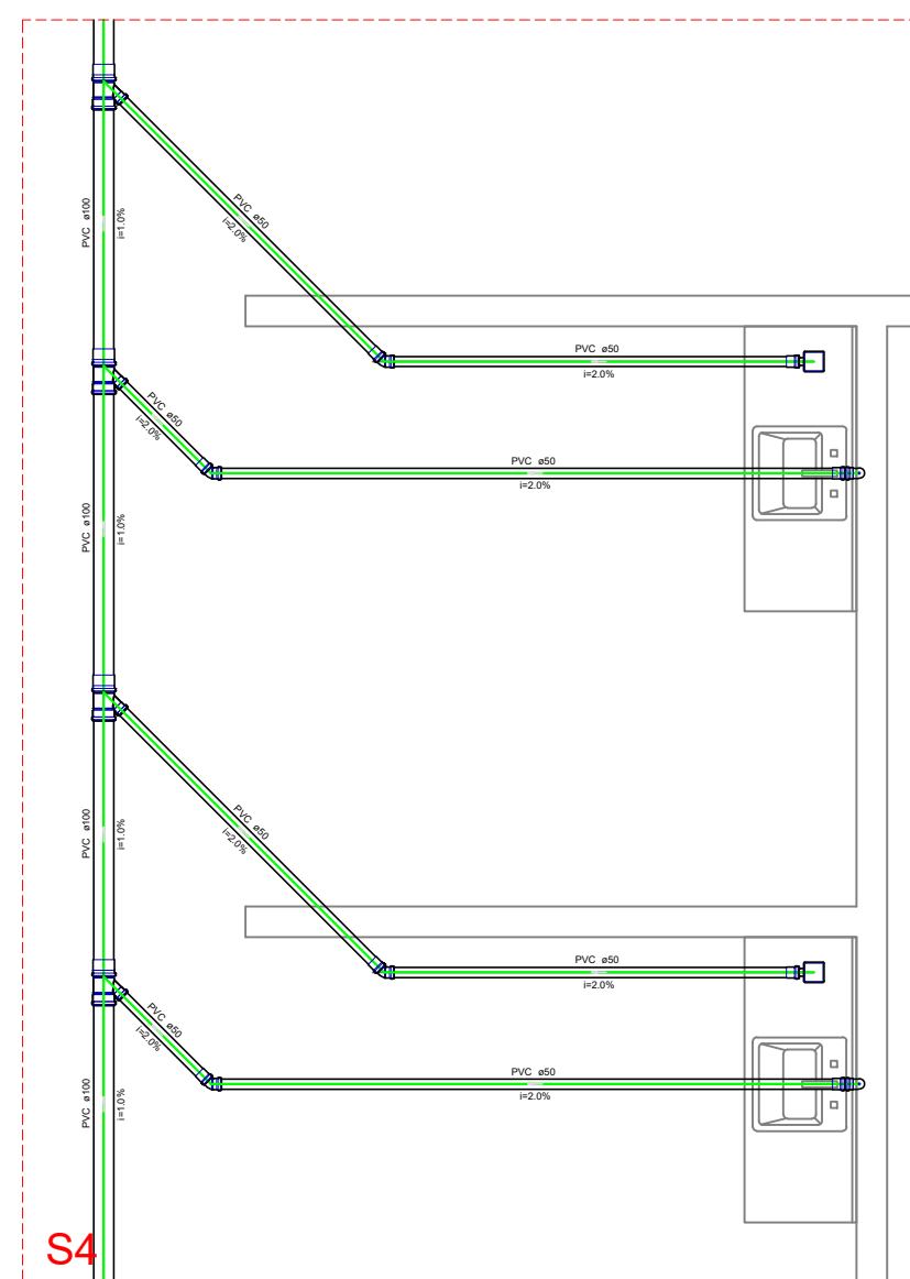
DETALHE S4
