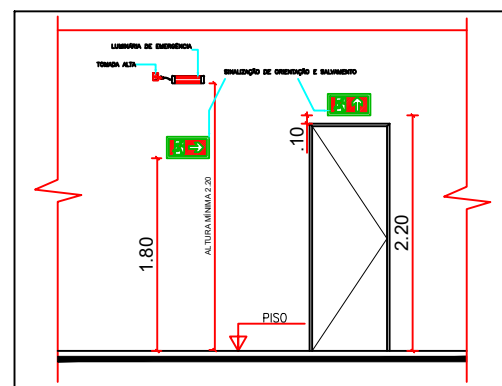
2/ESQ. SINALIZAÇÃO
