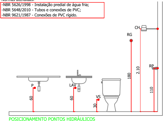
POSICIONAMENTO PONTOS HIDRÁULICOS
