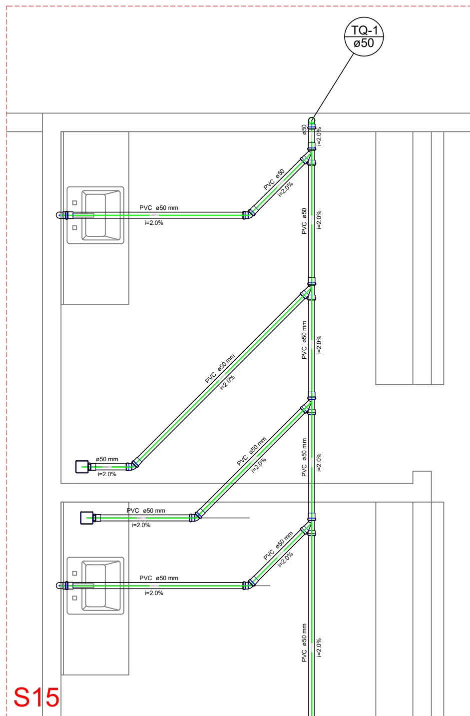
DETALHE S1
