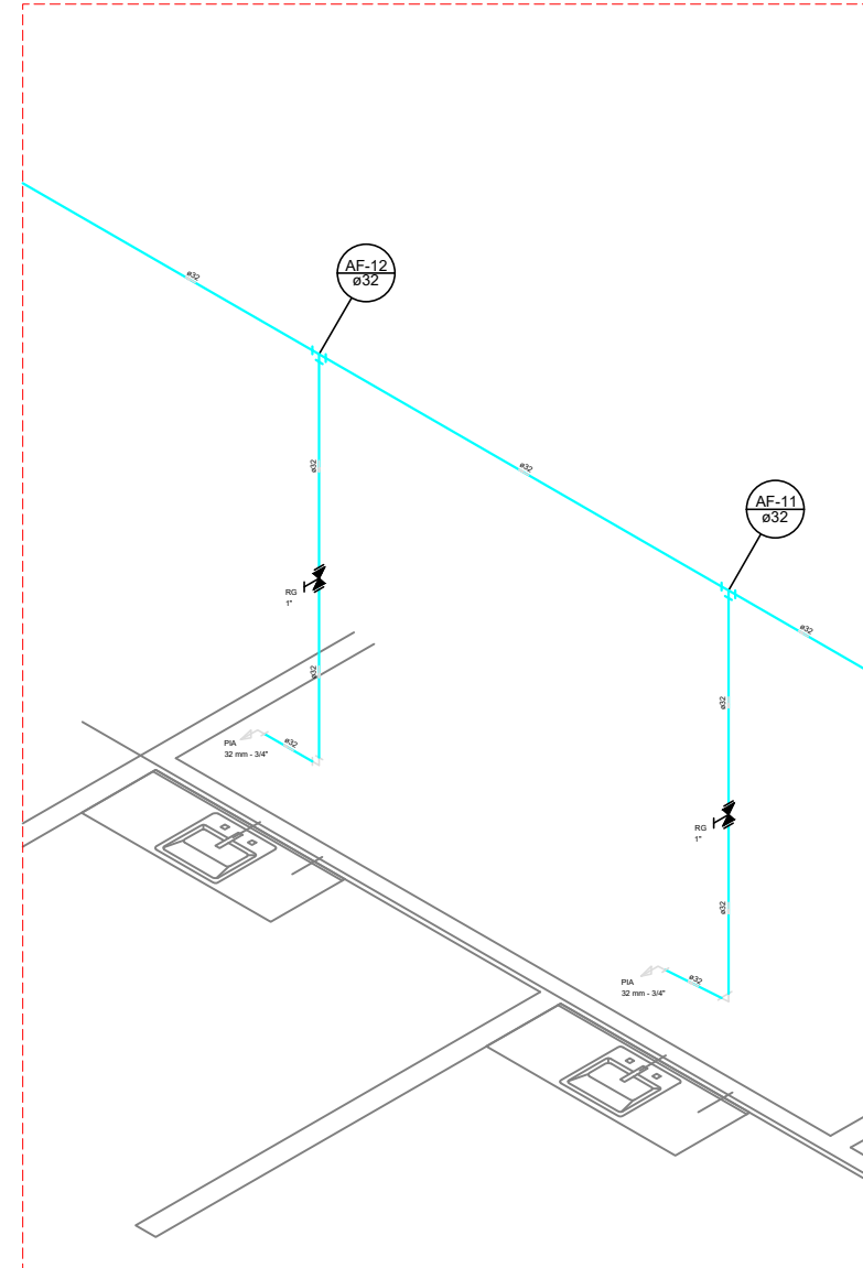
ISOMÉTRICO – H5 ESC. S/ESC
