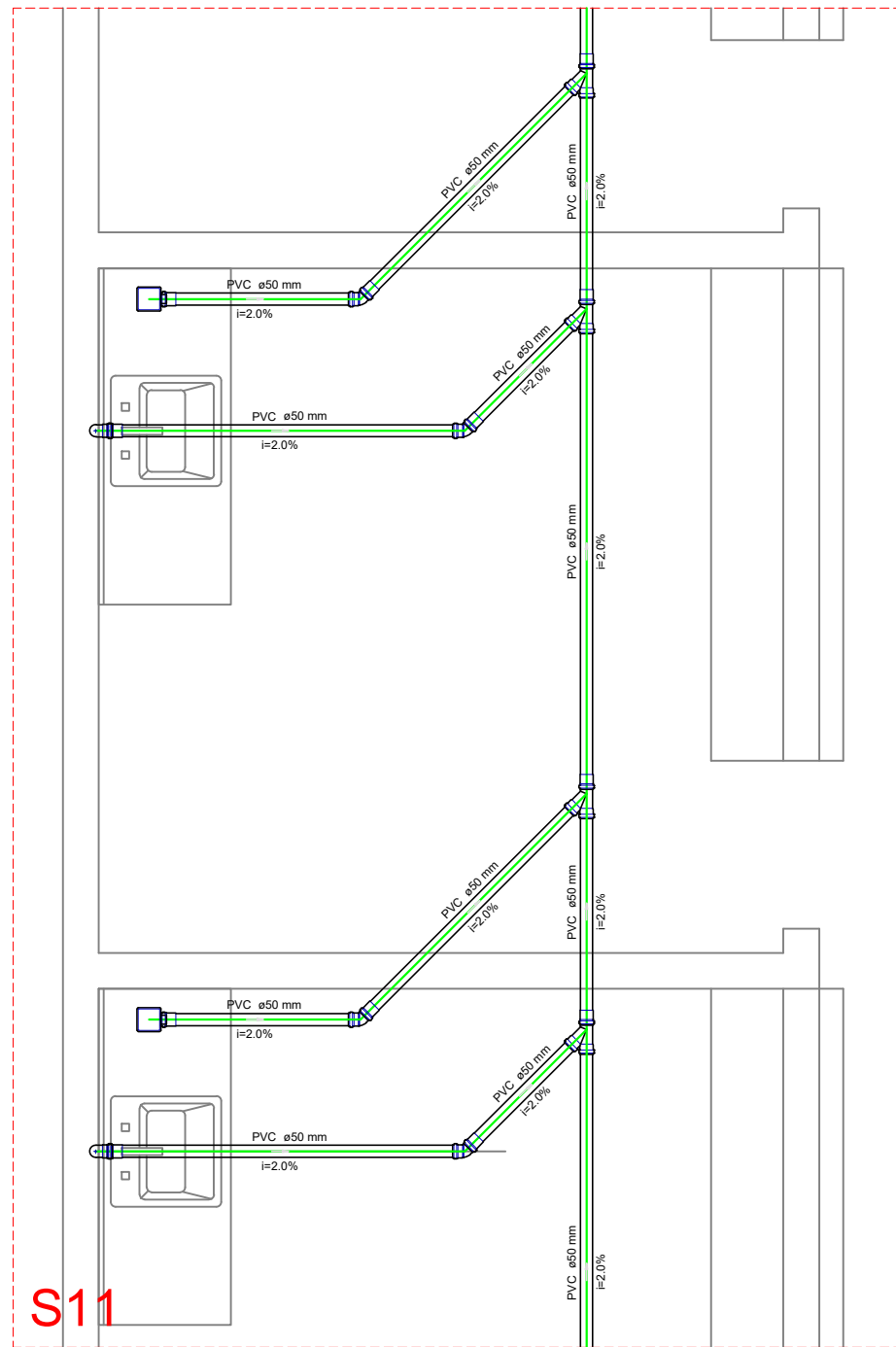
DETALHE S1
