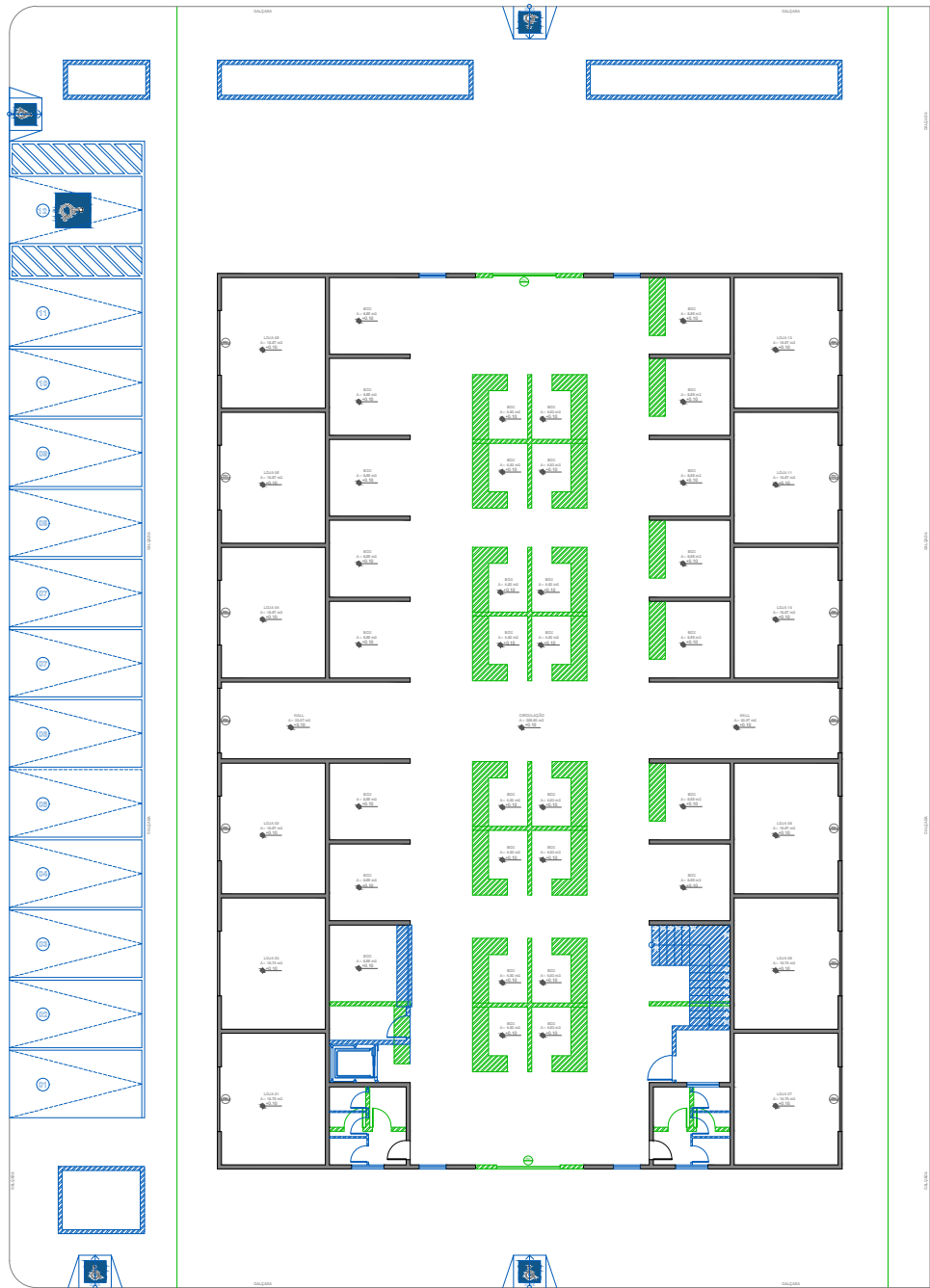
3 PLANTA DE DEMOLIÇÃO
