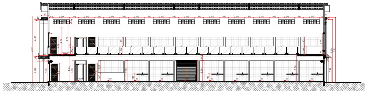
17 CORTE LONGITUDINAL CC 1:100
