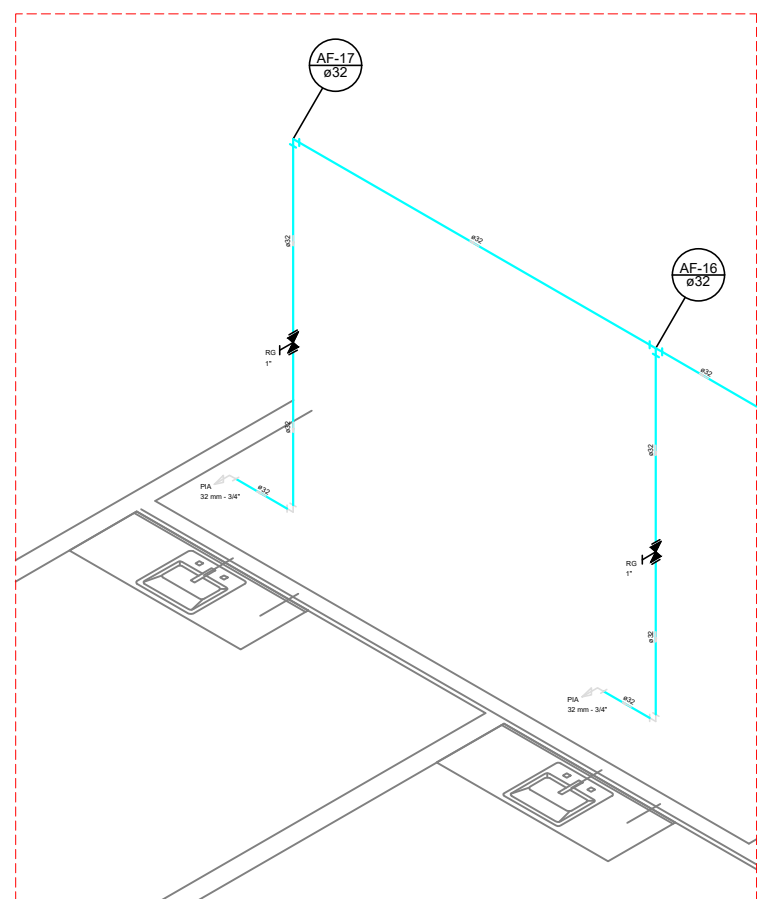
ISOMÉTRICO – H9 ESC. S/ESC
