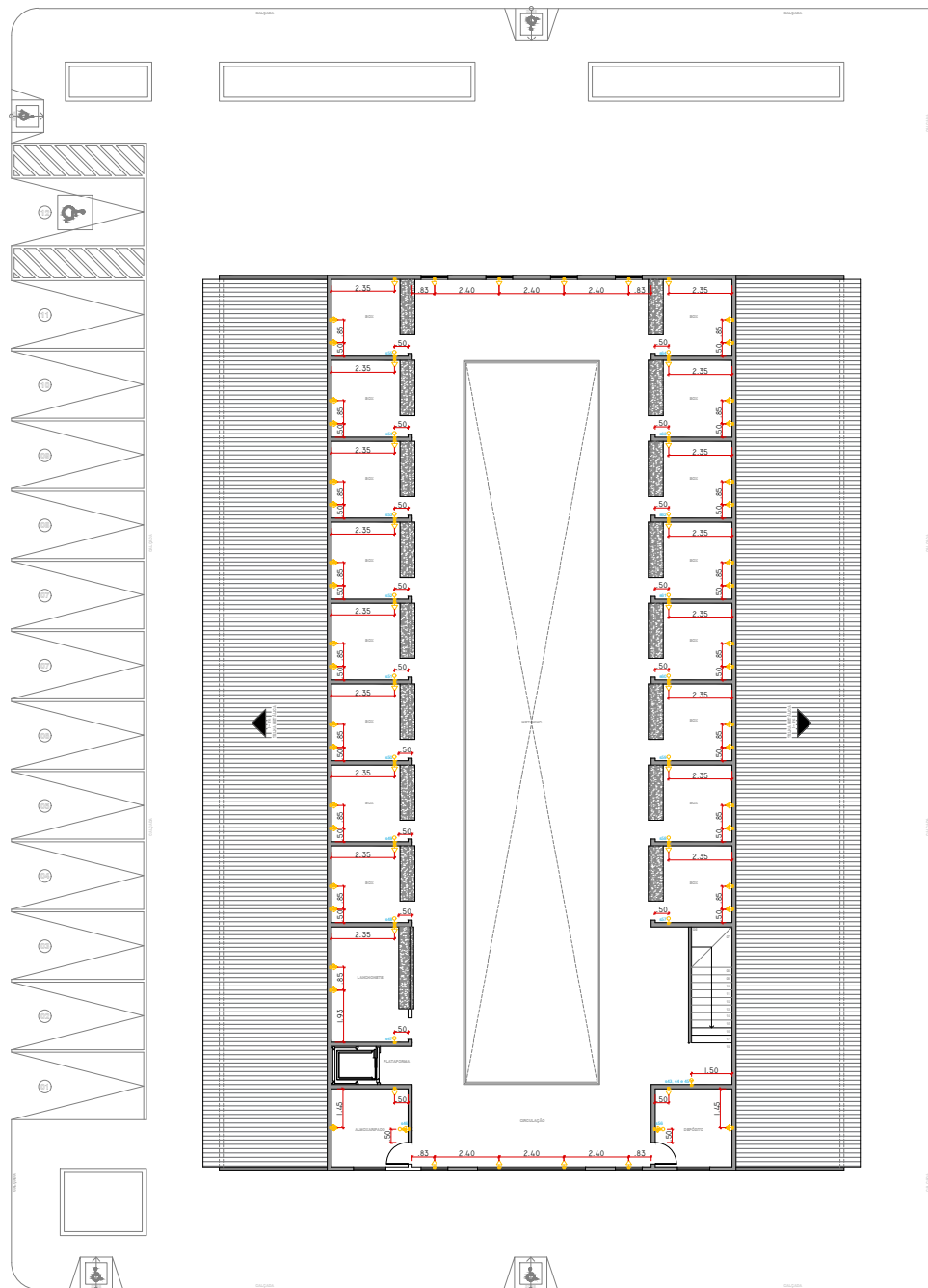
14 PLANTA DE PONTOS ELÉTRICOS 2 PAVIMENTO.
