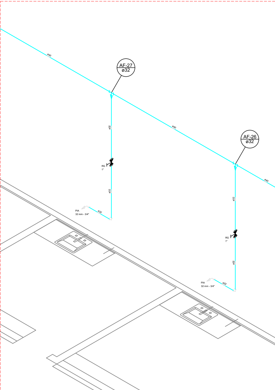
ISOMÉTRICO — H13 ESC. S/ESC
